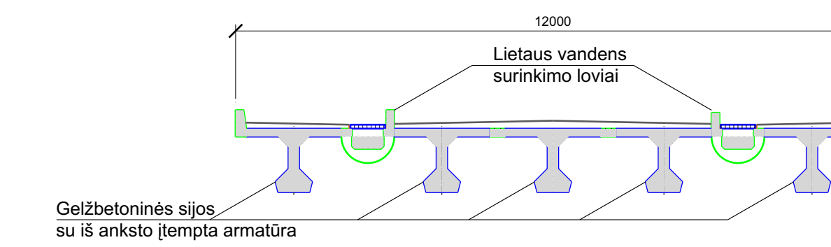
Konstruktinis pjūvis 2-2
