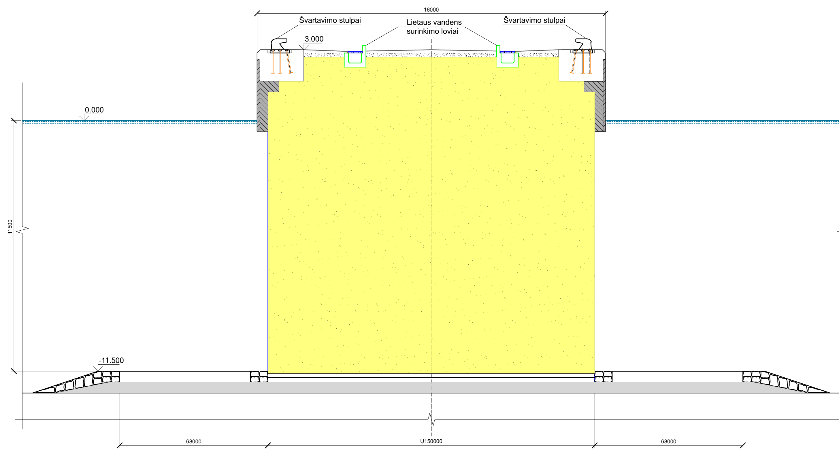
Konstruktinis pjūvis 1-1
